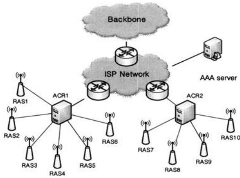
(그림 2) MBS상에서의 Single 과 Multi-RAS Access 방식
