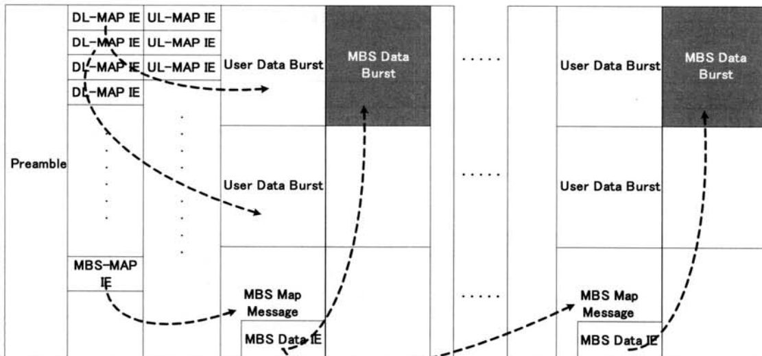
(그림 3) MBS Frame 구조
