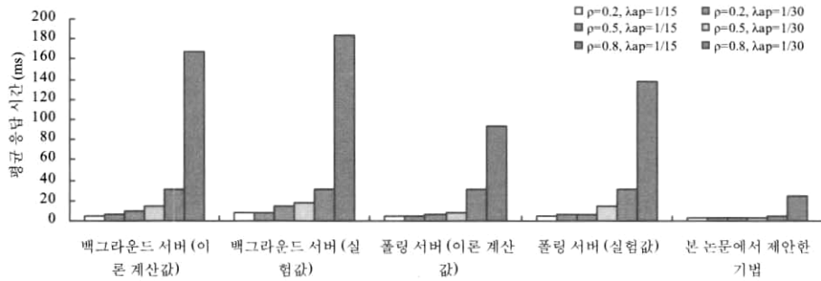
(그림 18) 비주기 태스크의 평균 응답 시간
