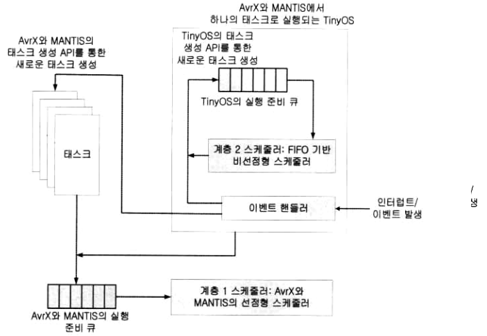
(그림 5) TinyOS를 태스크로 실행하는 AvrX와 MANTIS의 구조
