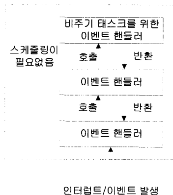
(그림 3) RTC (Run-To-Completion) 기반 비주기 태스크 구현 기법
