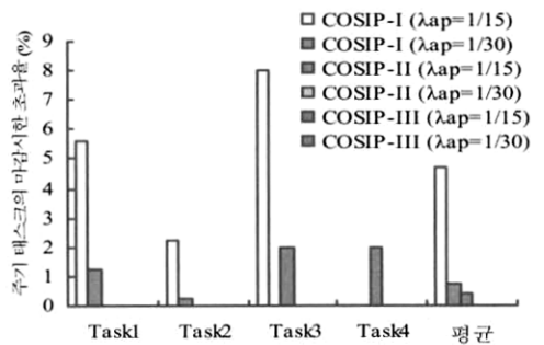
(그림 13) TA2에서 주기 태스크의 마감시한 초과율
