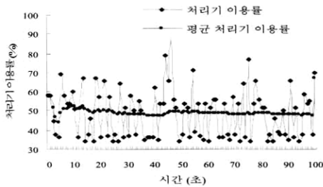
(그림 21) COSIP-II 모델
