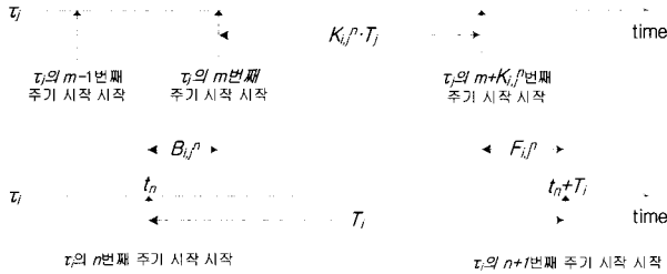
(그림 10) 주기 태스크 \tau_i 의 여유 시간
