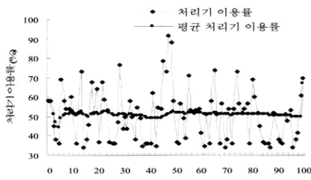
(그림 22) COSIP-III 모델
