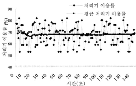
(그림 17) COSIP-III 모델
