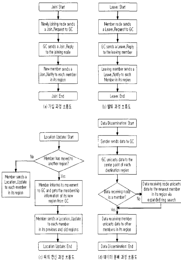
(그림 3) ROME 동작 과정 흐름도
