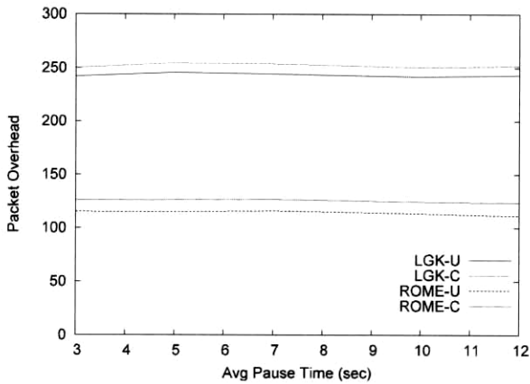
(그림 6) 평균 정지 시간의 변화에 따른 패킷 오버헤드
