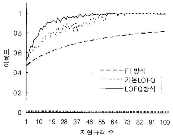
(그림 2) 대역폭 이용도(멀티미디어 응용)
