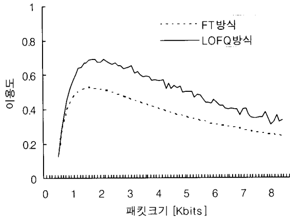
(그림 4) 유효 대역폭 이용도
