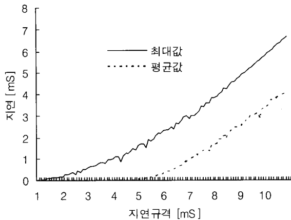
(그림 5) 레이턴시 측정 결과
