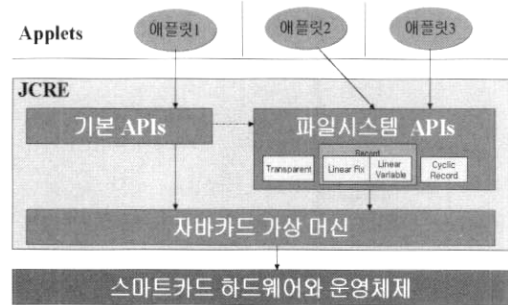
(그림 5) 파일시스템 API 구조
