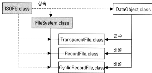
(그림 6) 파일시스템 API를 위한 각 클래스의 관계
