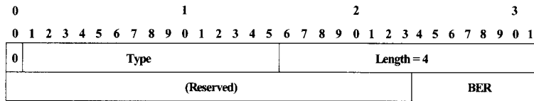
Type : 15bits, sub-TLV 타입을 나타낸다. Length : 16bits = 4 Reserved : 24bits, 0로 설정되어 수신시 무시되는 값이다. BER : 8bits, BER 표현의 역지수를 나타내며, BER이 10-X라면 BER 필드를 X로 설정한다.
