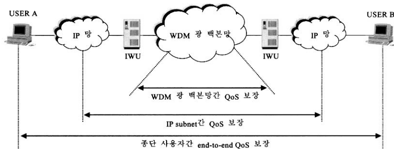
(그림 8) WDM 광 백본망을 통한 IP 서버넷의 QoS 보장
