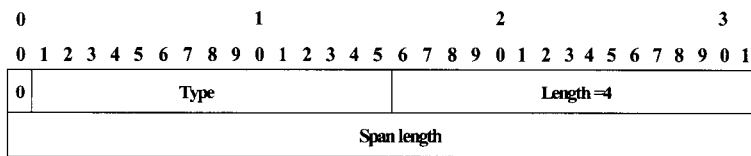
Type : 15bits, sub-TLV 타입을 나타낸다. Length : 16bits = 4 Span length : 32bits, WDM span의 총 길이(meters)로써, unsigned integer로 나타낸다.
