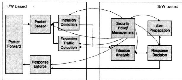
(그림 4) 보안 노드의 블록 다이어그램
