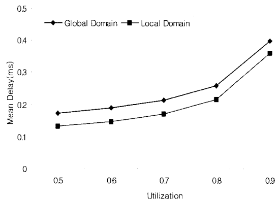
(그림 8) 네트워크 이용률에 따른 지연
