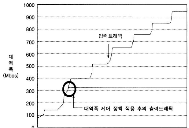
(그림 6) 대역폭 제어에 의한 과다트래픽 제어(320Mbps)
