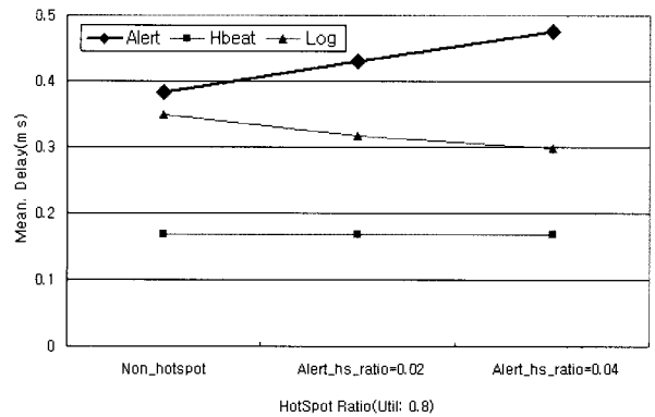
(그림 12) 경보 데이터의 핫 스팟 영향
