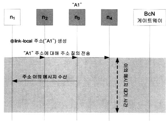
(그림 3) link-local 주소 할당 및 DAD 절차
