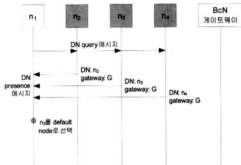
(그림 4) DN query/presence 메시지 및 DN 선택 절차
