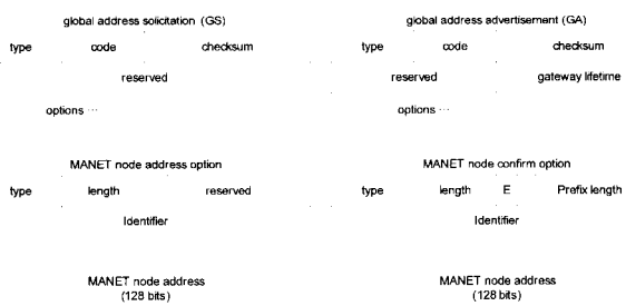
(그림 8) GS 및 GA 메시지 정의
