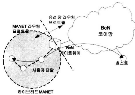
(그림 1) 하이브리드형 MANET 액세스 네트워크 모델
