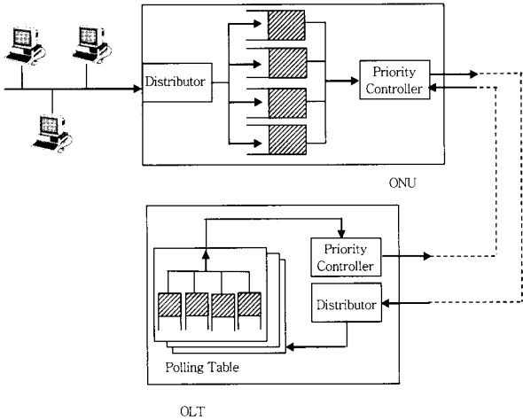
(그림 4) 제안된 DBA 방식의 기능 블록도
