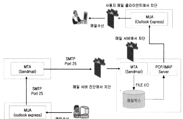
(그림 2) 정크 메일 대응시점에 따른 차단방법
