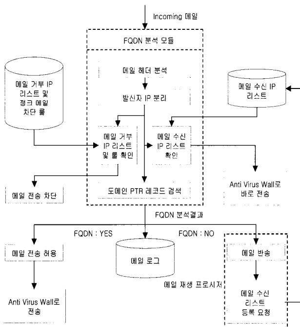
(그림 7) FQDN 확인을 이용한 정크메일 차단 모듈 구성도
