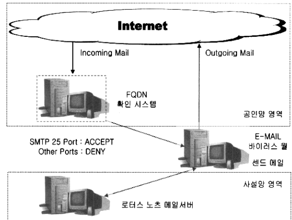
(그림 9) FQDN 확인을 이용한 개선된 정크메일 차단 시스템 구성
