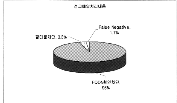
(그림 12) FQDN 확인을 이용한 정크메일 차단 결과 정크메일 처리내용
