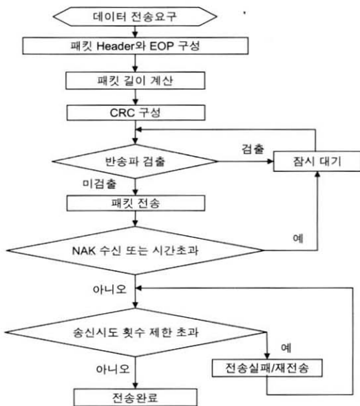
(그림 2) 무선모뎀 프로토콜의 패킷 송신 절차
