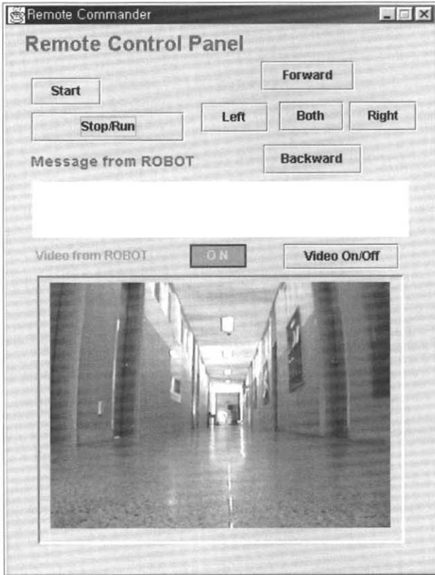
(그림 7) 제어 프로그램
