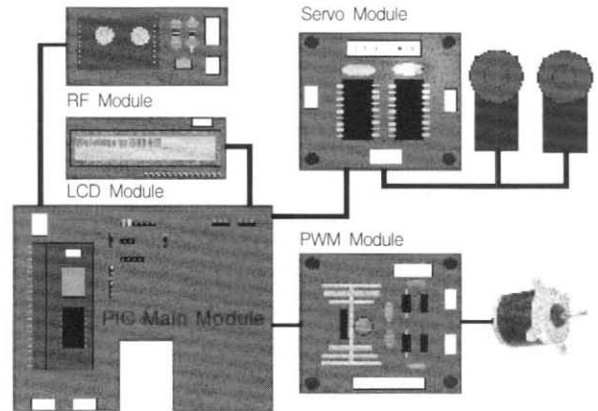
(그림 2) 로봇 제어 회로의 블록도
