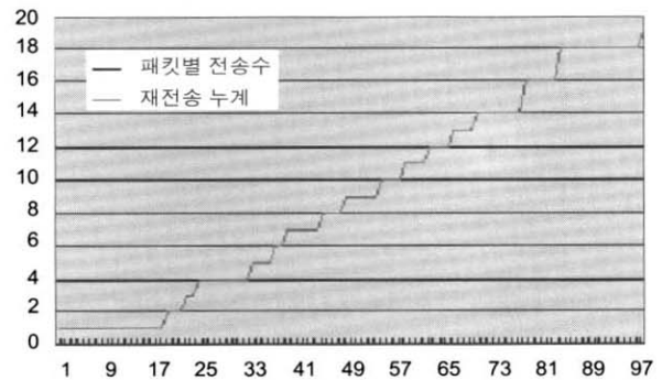
(그림 8) 패킷별 재전송 횟수의 누적표
