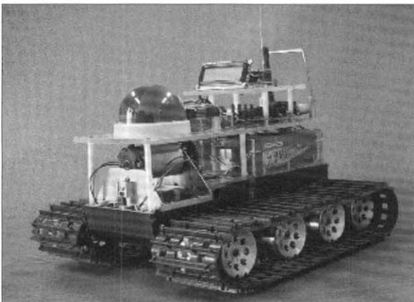
(그림 5) 실험에 사용된 로봇
