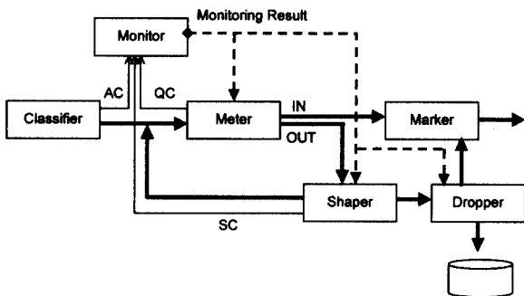
(그림 9) 제안하는 Traffic Conditioner 모델
