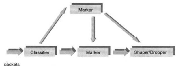
(그림 3) Traffic Conditioner
