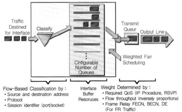
(그림 7) Weighted Fair Queuing
