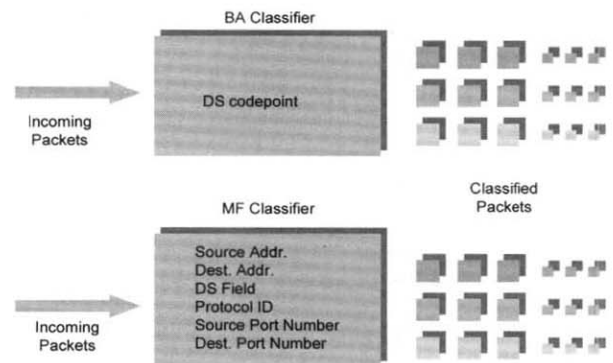
(그림 2) Classifier의 종류
