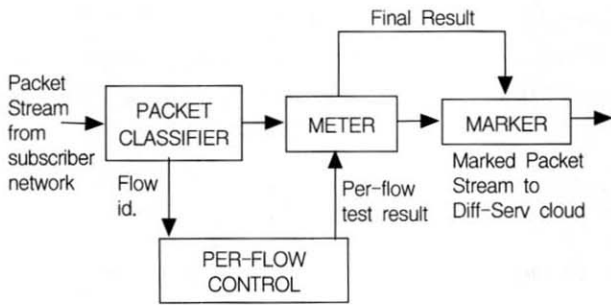
(그림 6) FM 블록도
