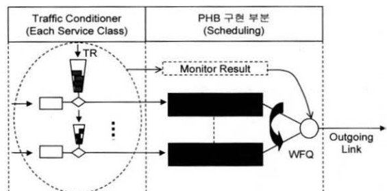
(그림 8) DS Node에서의 TC와 PHB구현의 관계
