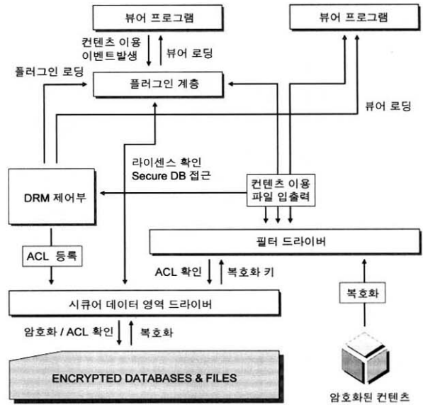
(그림 12) DRM 클라이언트 구성도
