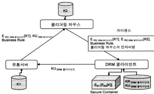
(그림 10) 라이선스 기반 암호화 키 전달 흐름
