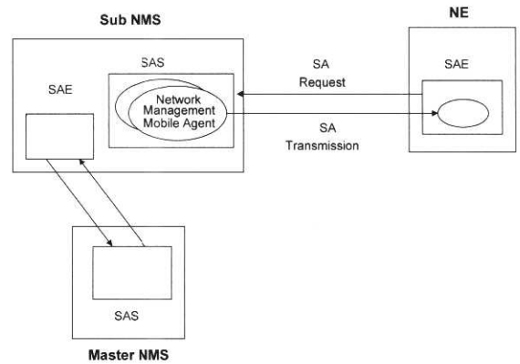
(그림 4) 이동 에이전트 시스템 구성
