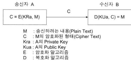
(그림 2) 전자서명 메커니즘
