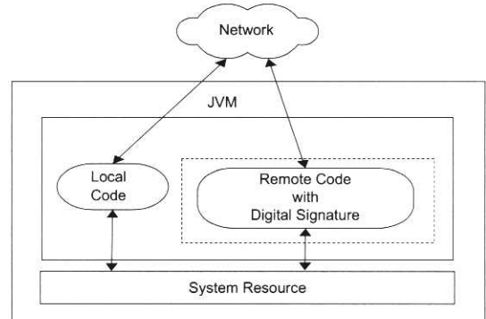
(그림 3) Signed Applet의 실행
