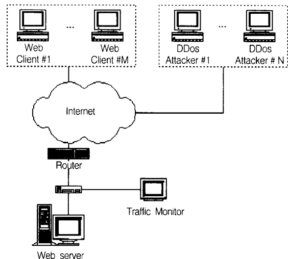
(그림 3) 실험을 위한 네트워크의 구성
