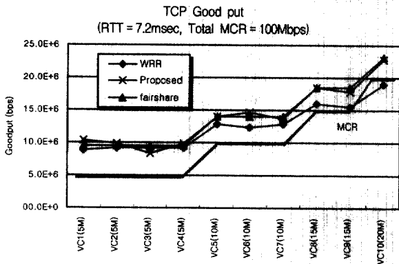
(그림 7) TCP의 Goodput(RTT = 7.2 msec, Total MCR = 100 Mbps)
