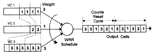
(그림 1) WRR 기법의 구조
