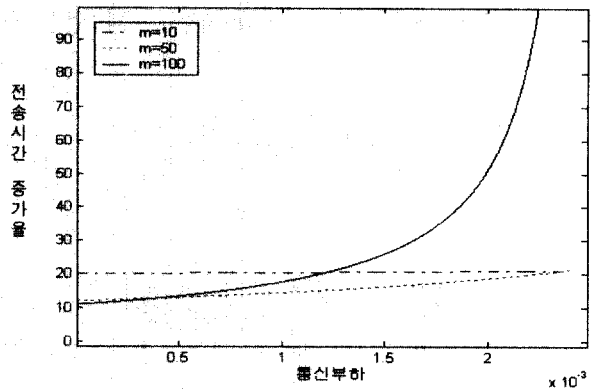
(b) m개의 패킷 전송시간 증가율 (그림 8) 통신 모델 (c)의 통신 부하에 따른 전송 시간 증가율
