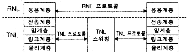
(그림 2) 통신관련 일반 프로토콜 스택 구조
