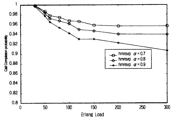
(그림 19) 성능 파라메타 ( \alpha = 0.7, 0.8, 0.9 )에 따른 호의 서비스 완료율
