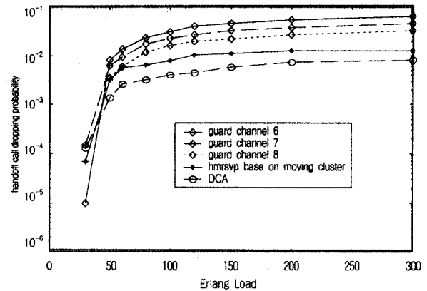
(그림 15) 핸드오프 호 손실율 / Erlang Load
