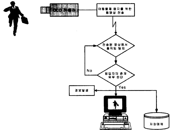
(그림 9) 무인감시장치의 움직임 탐지 구현의 구성도.
