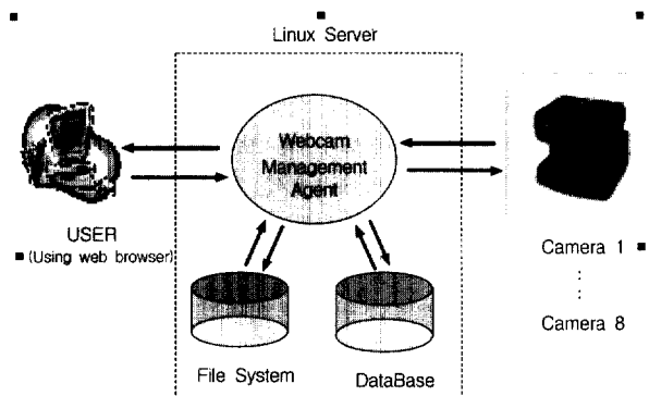
(그림 3) 제안된 웹캠 시스템의 개념적 구조
