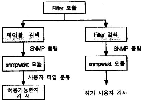
(그림 5) 포트 필터링 흐름도
