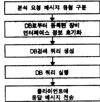
(그림 7) 누적 성능 분석 모듈 흐름도
