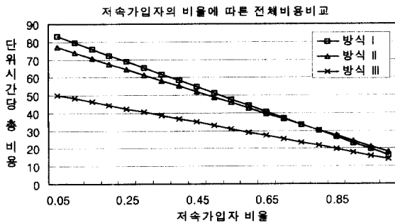
(그림 8) 저속가입자의 비율증가에 따른 영역관리 비용
