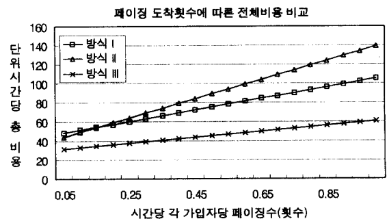
(그림 7) 페이징 발생횟수에 따른 영역관리 비용
