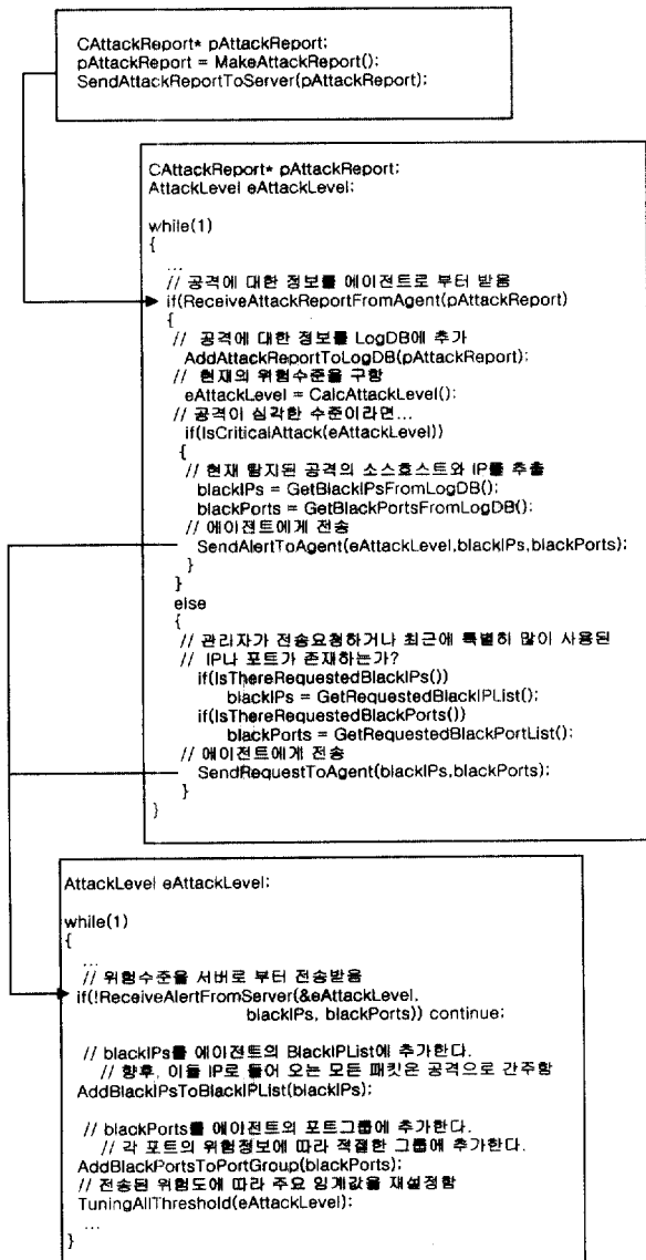
(그림 4) 에이전트와 서버사이의 계층적 탐지알고리즘
