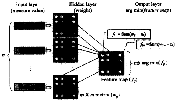
(그림 3) SOM layer
