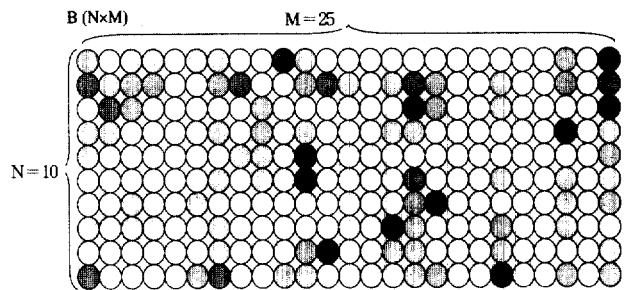
(그림 13) HMM model 예 (root에 대한 B행렬 값)
