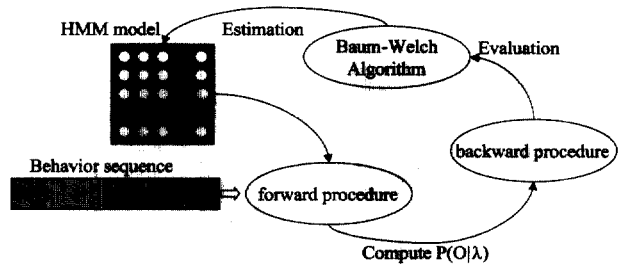
(그림 6) 정상행위 모델링 모듈 동작 시나리오
