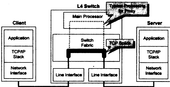
(그림 2) TCP Splicing 기능을 탑재한 디스패칭 시스템의 블록 개요도
