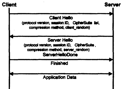
(b) 간이 핸드셰이크 과정
