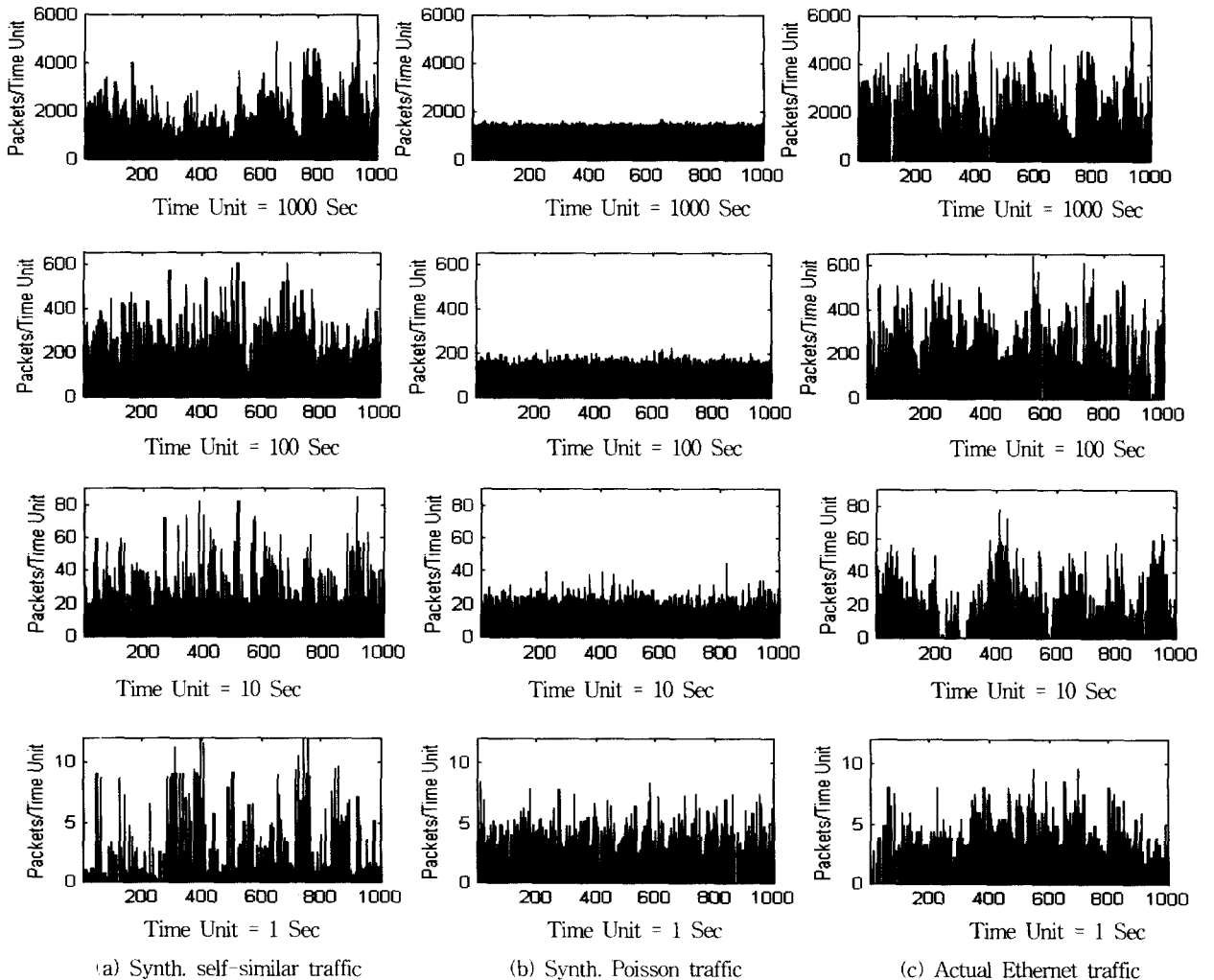
(그림 4) Aggregation 레벨에 따른 실제 트래픽과 합성 트래픽의 비교
