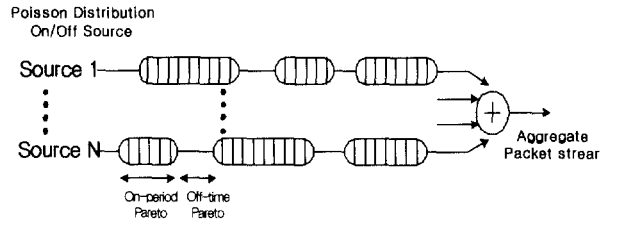
(그림 3) Poisson 트래픽 발생기의 블록 다이어그램
