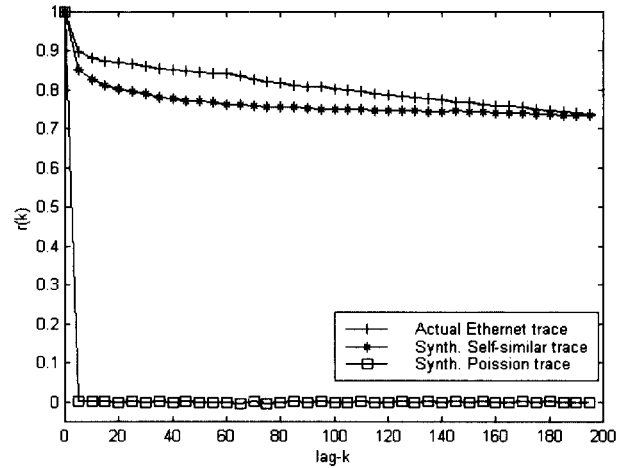
(그림 5) 시차(lag-k)에 따른 자기상관함수
