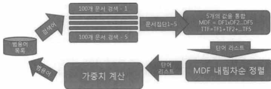
(그림 1) 범용어 자동 수집 알고리즘
