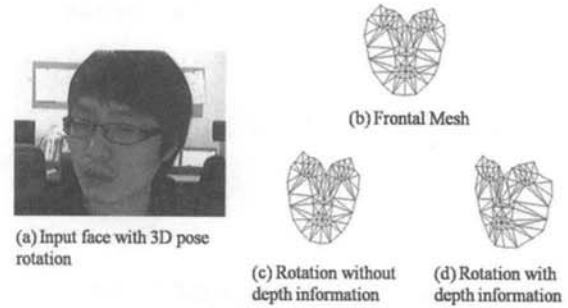
(그림 6) 깊이 정보를 포함한 매쉬와 포함하지 않은 매쉬의 3차원 회전 변환 예
