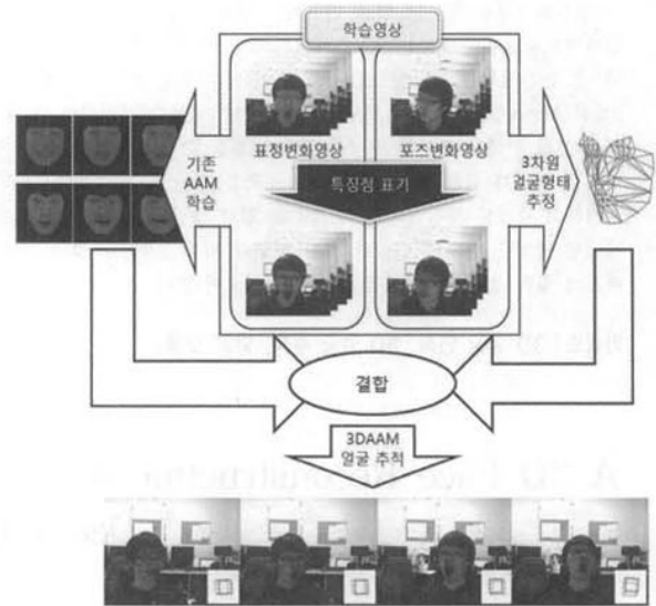
(그림 1) 제안된 시스템의 학습 모듈
