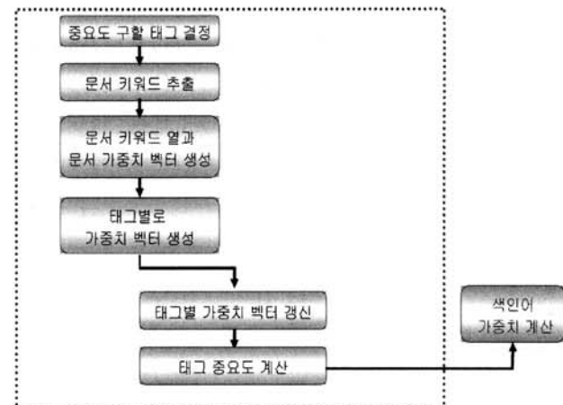
(그림 1) 태그별 색인어 가중치 결정 흐름도
