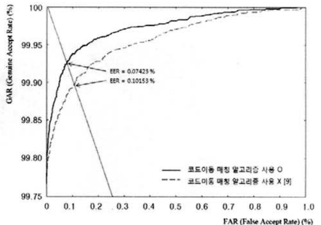
(그림 14) 코드 이동 매칭 알고리즘의 사용 및 미사용에 대한 ROC 곡선
