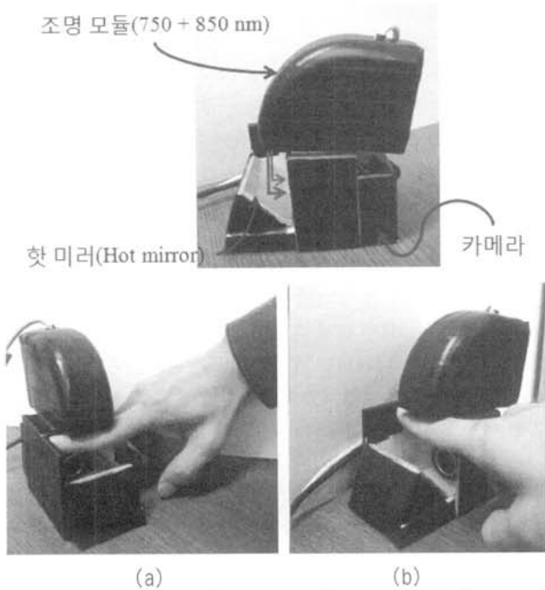
(그림 1) 제안하는 손가락 정맥 영상 취득 장비의 견본(prototype) : (a) 제안하는 장비 (b) 장비를 사용하는 예[11]
