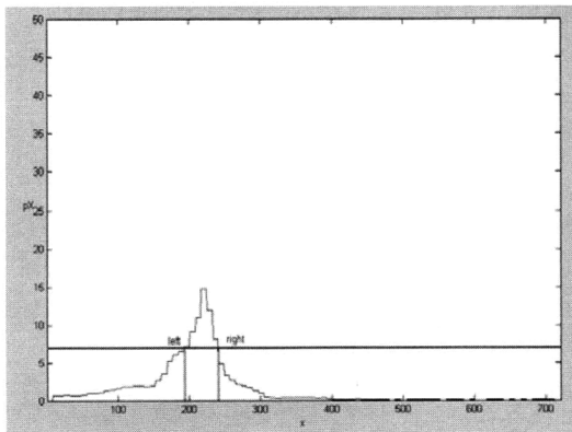
(a) PX(x,t)
