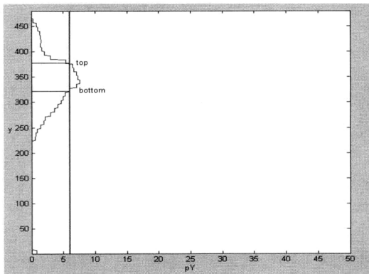
(b) PY(y,t)
