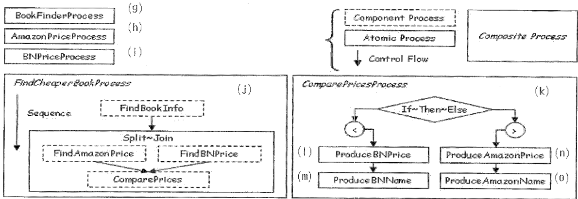
(그림 10) FindCheaperBookProcess 제어 구조
