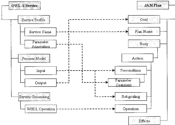
(그림 6) 기본 서비스 명세와 JAM 계획 명세 비교
