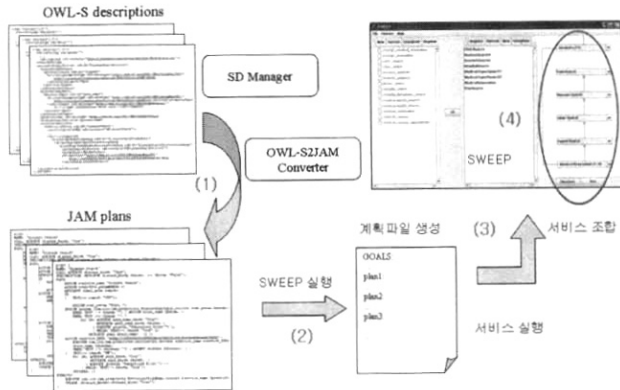
(그림 12) 조합과 실행 과정
