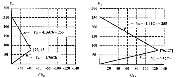
(그림 6) R 영역에서 휘도와 CbCr 색차 신호의 관계 그래프 (Figure 6) Luminance(Y) and Chrominance(CbR, Cr) vector relationship in R section
