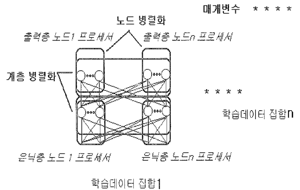
(그림 1) 신경망 병렬화의 수준
