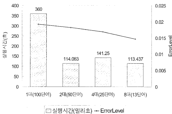
(그림 12) 링 네트워크위상에서 학습데이터 병렬화를 수행한 결과 차트
