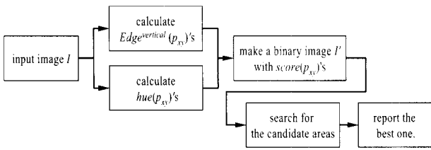
(그림 4) 번호판 영역 분할 알고리즘
