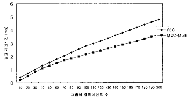
(그림 6) 평균 지연시간
