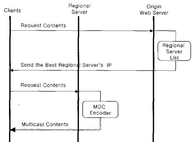
(그림 2) 지역서버에 의한 전송과정
