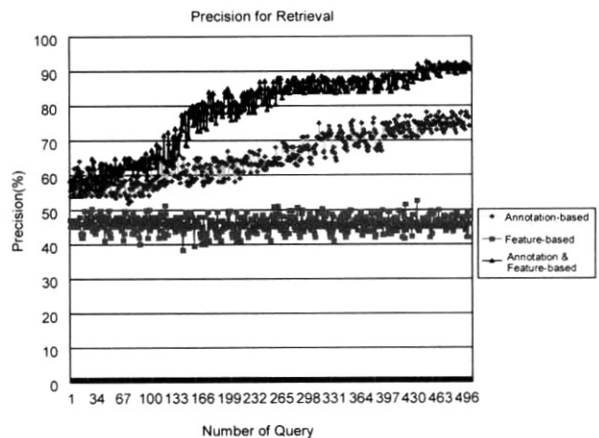
(그림 6) 제안 시스템의 검색 정확도
