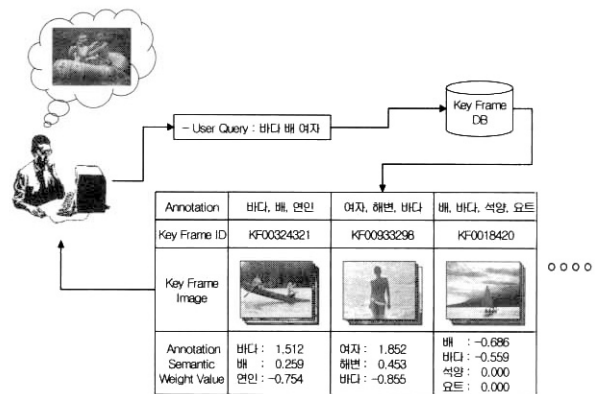
(그림 3) 키 프레임 주석 및 의미 가중치
