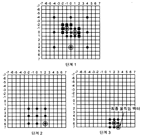
(그림 3) 새로운 3단계 탐색 기법(NTSS)
