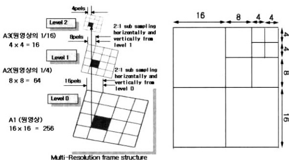
(그림 4) 다중해상도(MR : Multi Resolution)
