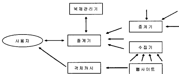
(그림 2) Harvest 구조
