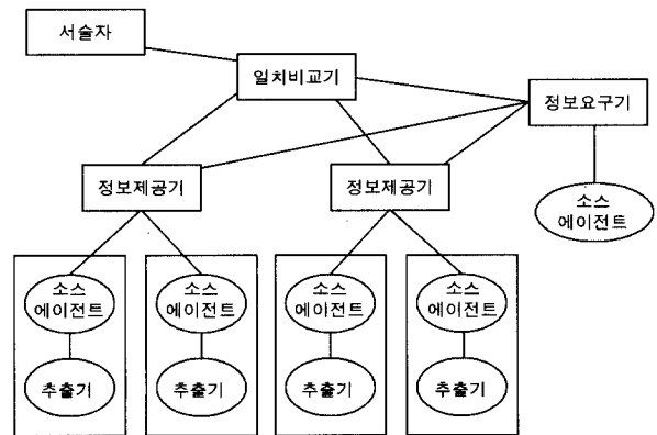
(그림 3) 웹에서 분산검색을 위한 멀티에이전트 구조
