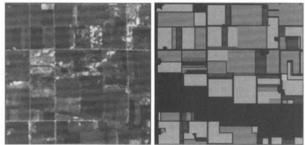
(그림 5) 4, 3, 2밴드를 RGB로 표현한 영상과 실측데이터
