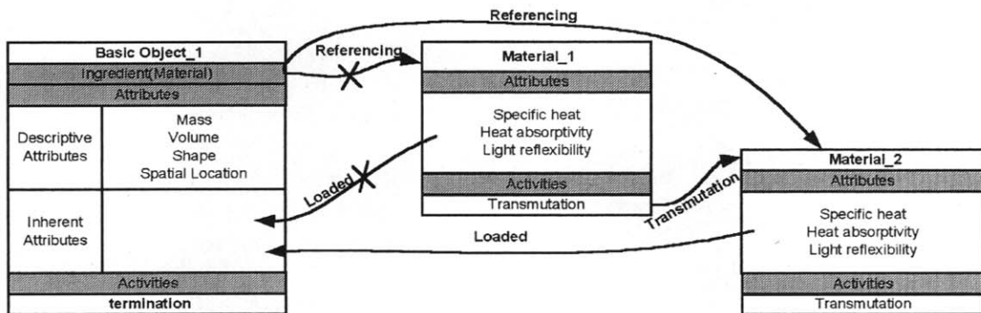
(그림 9) Ingredient의 상태 변화에 의한 Basic Object의 변화
