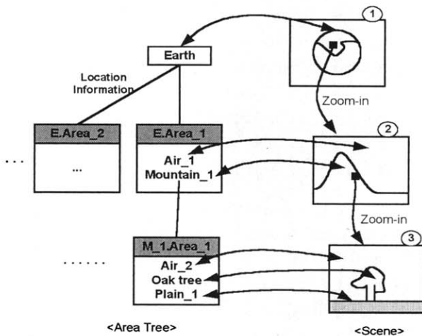
(그림 1) Area tree와 장면사이의 관계
