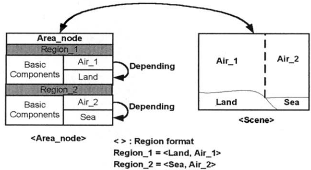
(그림 2) Area_node에서 지역 형성
