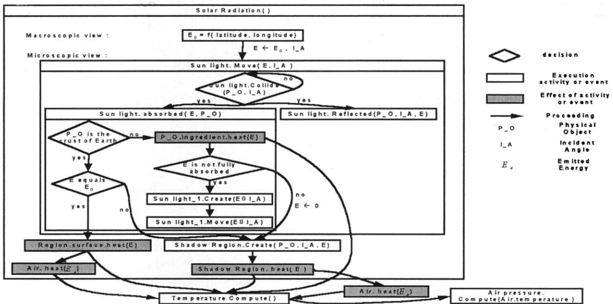
(그림 3) 태양 복사 이벤트의 과정
