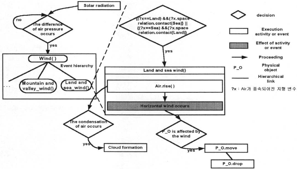
(그림 7) Wind Event Hierarchy 구조와 이벤트 진행과정의 예
