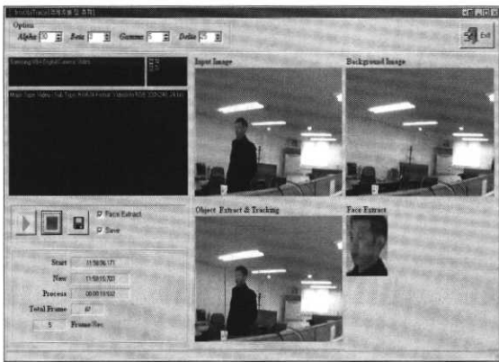
(그림 12) 실시간 객체 추적 및 얼굴 영역 추출 시스템
