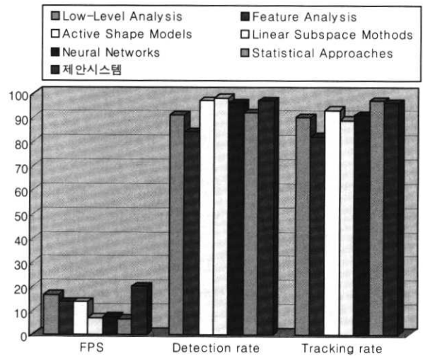
(그림 16) 시스템 성능 비교
