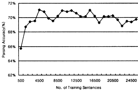
(그림 4) 평균 파싱 정확도 변화
