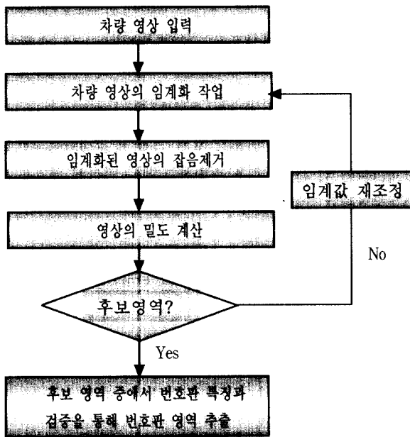
(그림 2) 차량 번호판 추출 구성도
