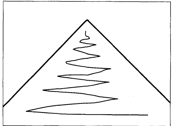
(그림 10) 관심영역결정
