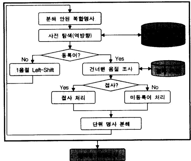
(그림 1) 복합명사 분해 흐름도
