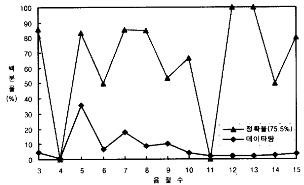
(그림 6) 파생어 분해 정확율
