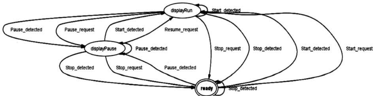
(그림 3) Main Automata
