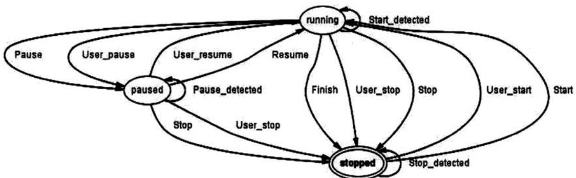
(그림 2) Simulink 모델 오토마타
