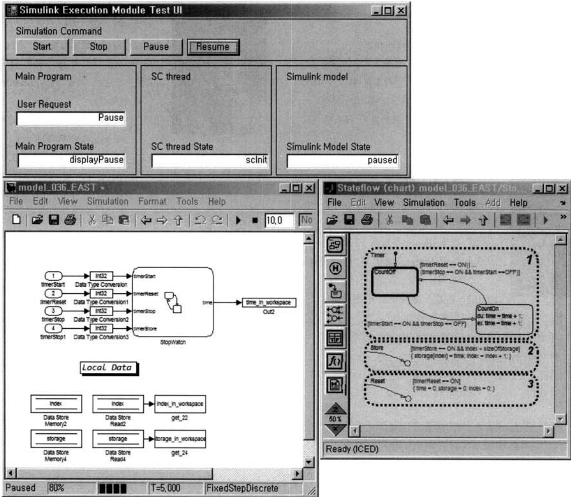
(그림 16) 테스트 프로그램과 예제 모델
