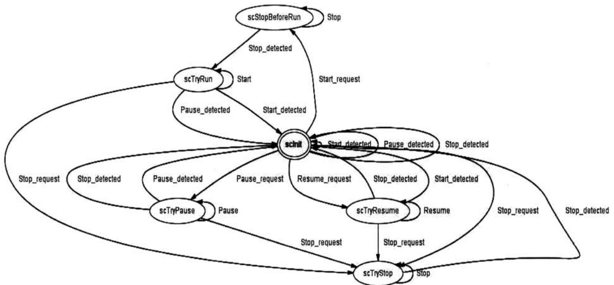
(그림 4) SC 스테드 오토마타
