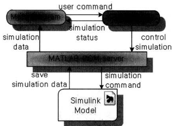
(그림 1) Simulink 실행 모듈
