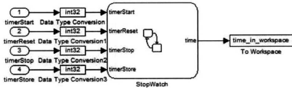
(그림 12) Simulink 모델 시뮬레이션 출력 저장
