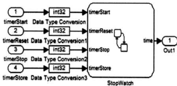
(그림 10) 스톱워치 예제 모델
