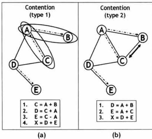
(그림 3) 페어 레지스터 할당 시 경쟁 상황
