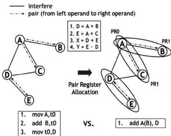
(그림 1) 페어 레지스터 할당 기본 개념도
