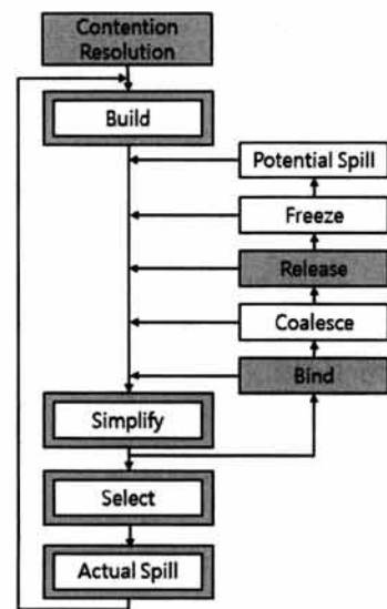
(그림 2) 페어 레지스터 할당 알고리즘 흐름도
