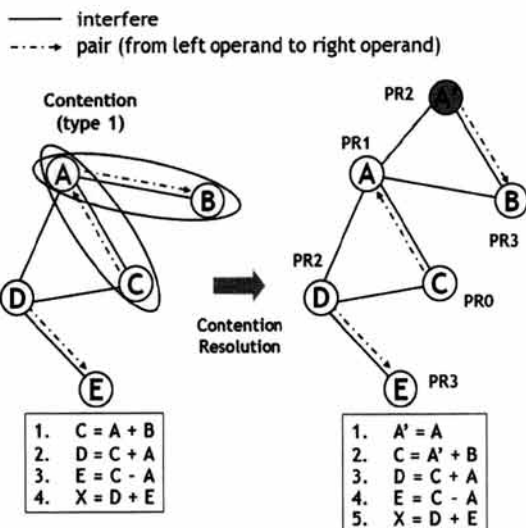
(그림 4) 경쟁 상황 1의 해결 과정
