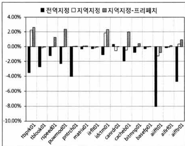
(그림 8) 페어 레지스터 지정 방식에 따른 실행 명령어 수의 감소 비율
