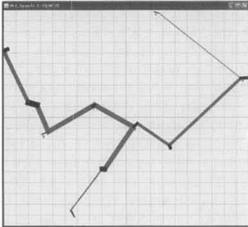
(그림 3) 최소 신장 트리를 이용한 가중치 입력 선분 연결 (비용=467.1679)
