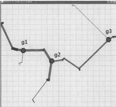
(그림 5) EGOSST를 이용한 가중치 입력 선분 연결(비용=421.9342)
