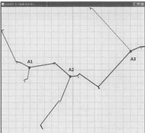
(그림 7) 입력 선분 10, 최대 가중치 5, 그리드 정밀도 0.1 환경에서의 EGOSST 생성 결과 (비용=171.7382)
