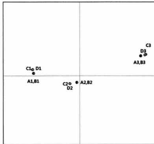
(그림 11) 각 조건에 따라 생성된 연결 지점의 위치 비교
