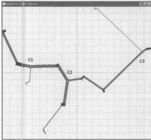
(그림 9) 입력 선분 10, 최대 가중치 20, 그리드 정밀도 0.1 환경에서의 EGOSST 생성 결과 (비용=421.9595)
