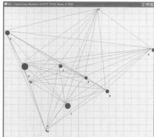
(그림 2) 가중치 입력 선분의 노드 변환 및 완전 연결 생성
