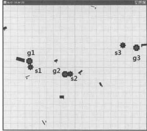
(그림 6) 스타이너 포인트와 GOSST 포인트의 위치 비교
