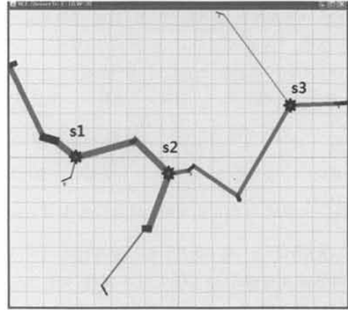
(그림 4) 근사 스타이너 최소 트리를 이용한 가중치 입력 선분 연결 (비용=437.8393)
