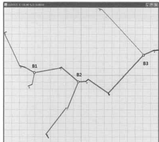
(그림 8) 입력 선분 10, 최대 가중치 5, 그리드 정밀도 0.001 환경에서의 EGOSST 생성 결과 (비용=171.7244)
