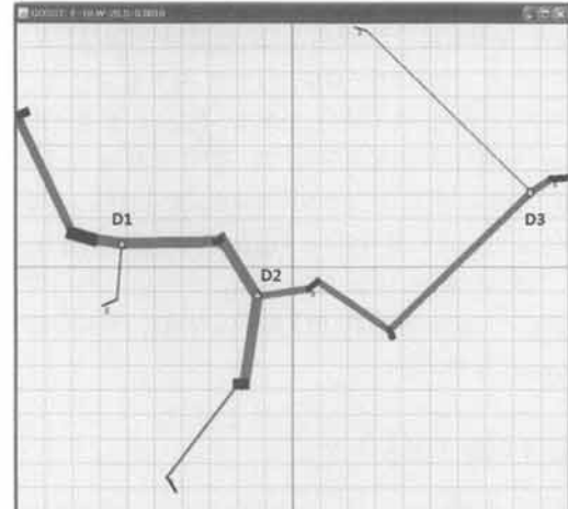
(그림 10) 입력 선분 10, 최대 가중치 20, 그리드 정밀도 0.001 환경에서의 EGOSST 생성 결과 (비용=421.9342)
