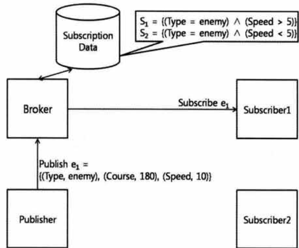
(그림 3) Broker의 이벤트 매칭
