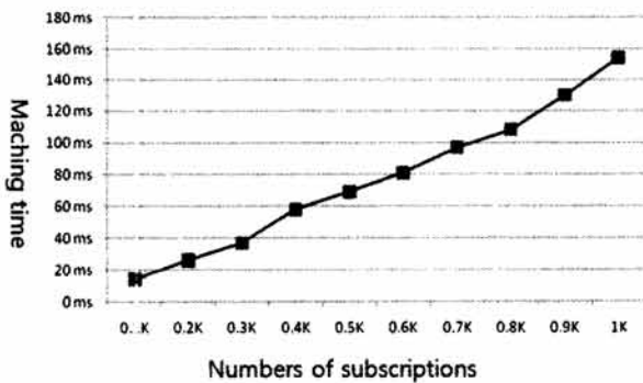
(그림 11) 순차검색을 통한 매칭시간 결과
