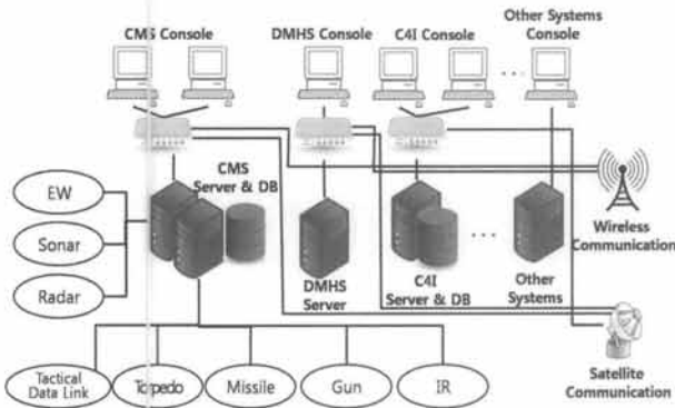
(그림 6) 함정 시스템의 시스템 구성
