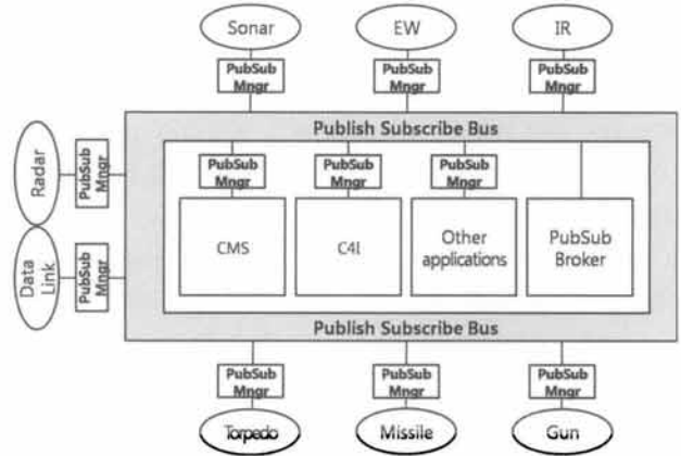
(그림 7) 제안 정보교환 아키텍처
