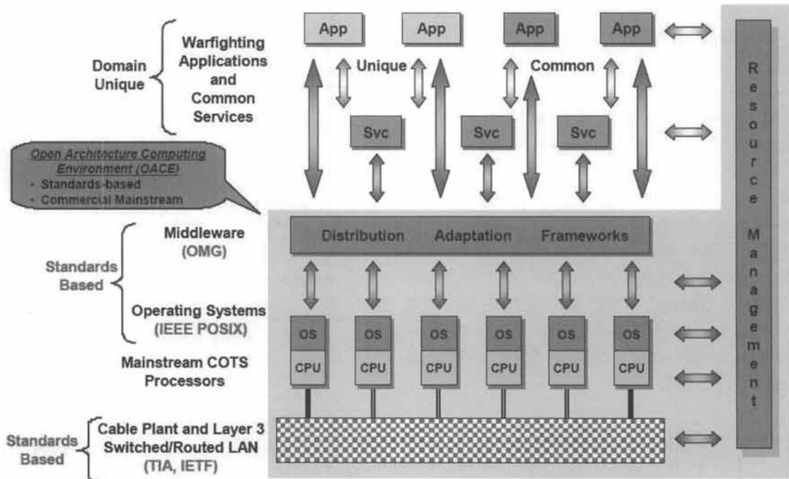
(그림 4) 개방형구조(OA) 계층[4]
