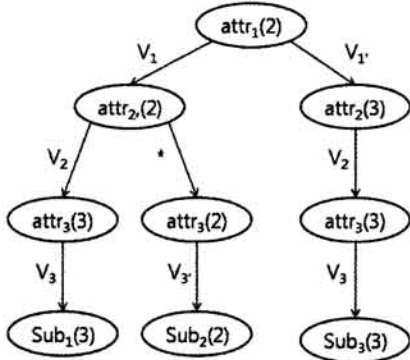
(그림 13) 제안 이벤트 매칭 트리
