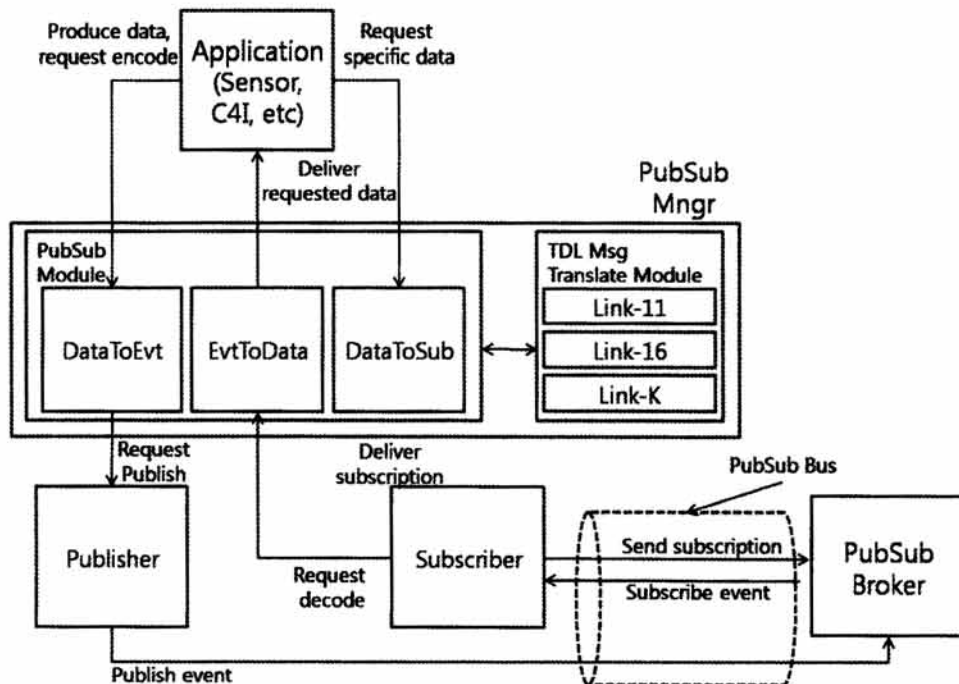
(그림 9) PubSub 매니저 역할
