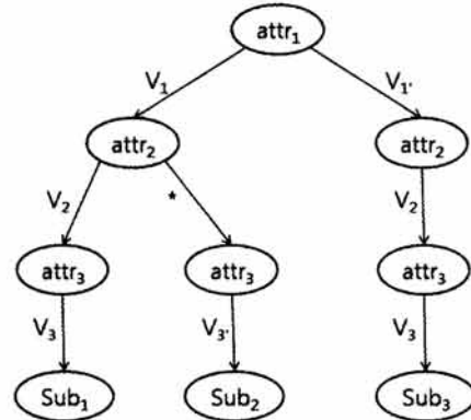
(그림 12) 이벤트 매칭 트리
