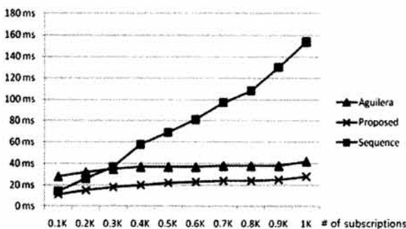
(그림 18) 순차검색과 매칭 트리 알고리즘 매칭 시간 비교
