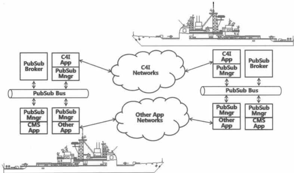
(그림 8) 기존 애플리케이션 네트워크를 통한 정보교환
