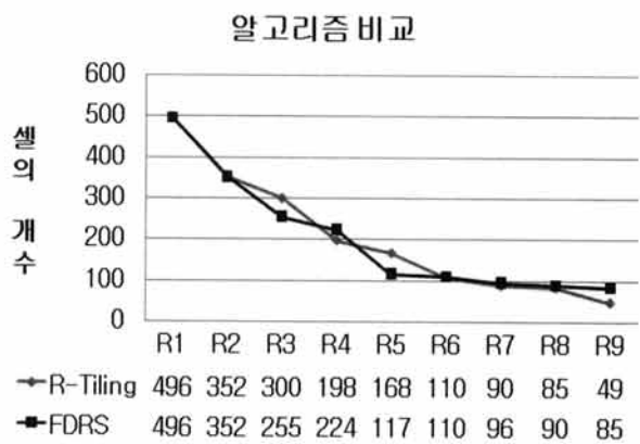
(그림 10) 오차 발생 map에서 두 알고리즘의 R1~R9까지의 크기(단위는 사각형의 크기)
