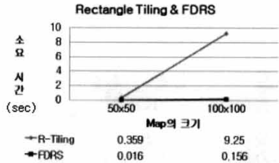
(그림 6) 실제 환경에서의 map크기에 따른 알고리즘 비교
