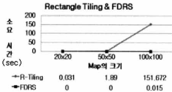
(그림 4) 일정한 수의 장애물에서 map의 크기에 따른 알고리즘 비교
