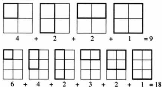
(그림 1) Rectangle Tiling의 원리(그림 출처: http://mathworld.wolfram.com/RectangleTiling.html )
